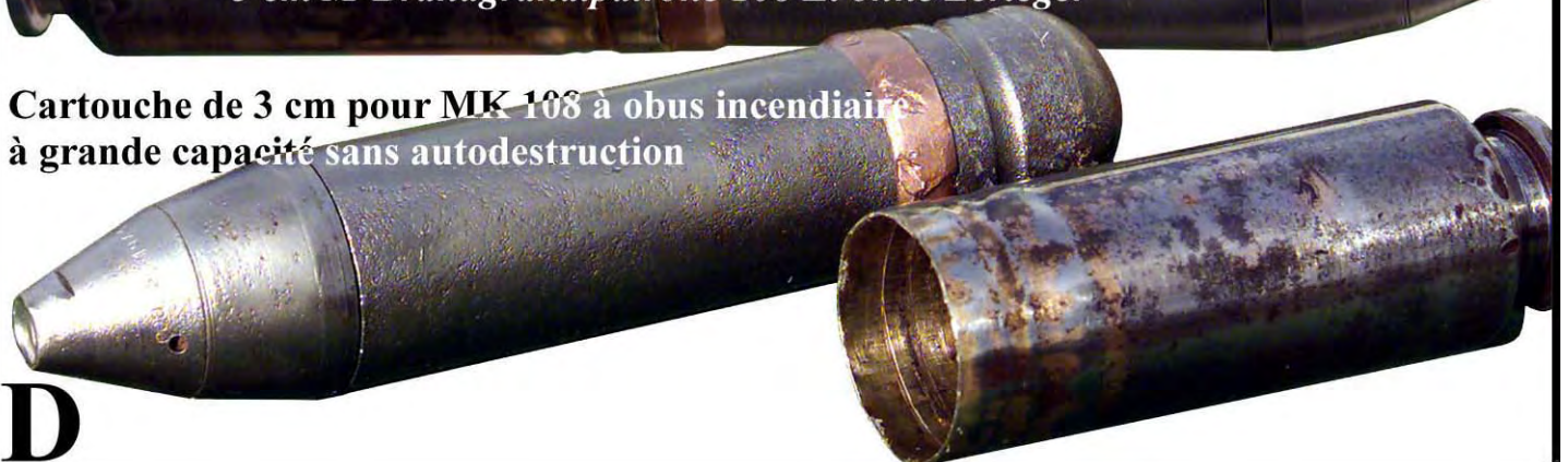
3 cm M-Brandgranatpatrone 108 El ohne Zerleger
