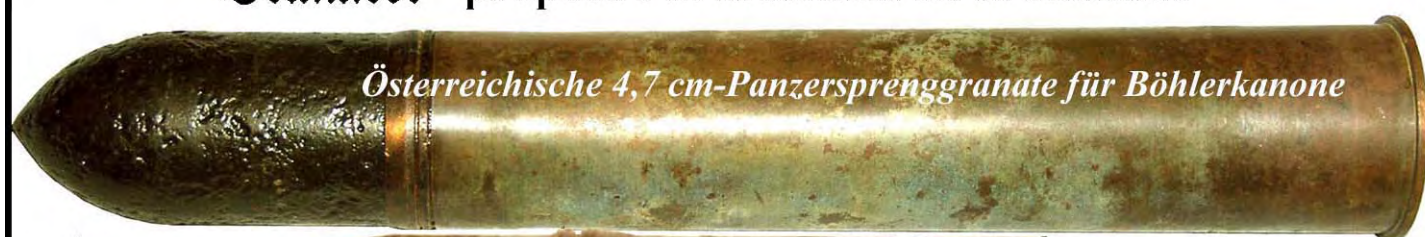
Obus de rupture autrichien de 4,7 cm pour canon Böhler
