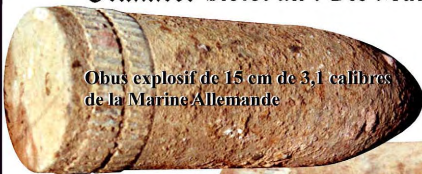
15 cm-Sprenggranate L/3,1 der Deutschen Marine
