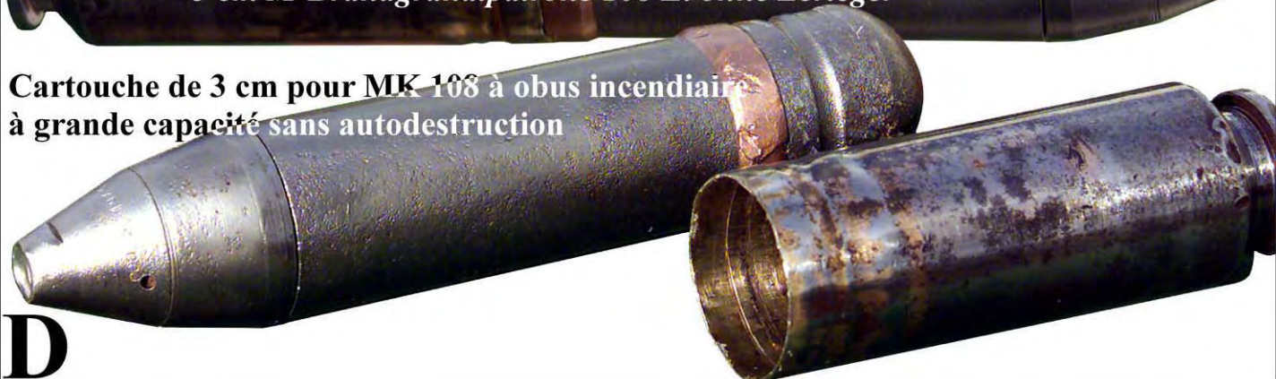
3 cm M-Brandgranatpatrone 108 El ohne Zerleger
